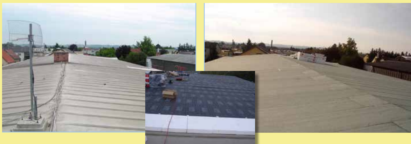
Falzblechdachsanieierung mit zusätzlicher Wärmedämmung
